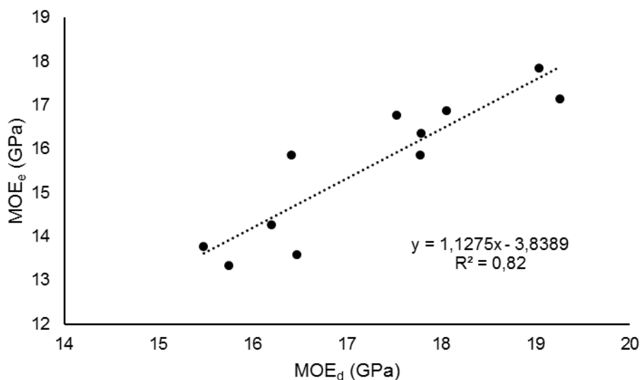
Figura 1. Modelo de regressão para os módulos de elasticidade dinâmico (MOE d ) e estático (MOE e )
