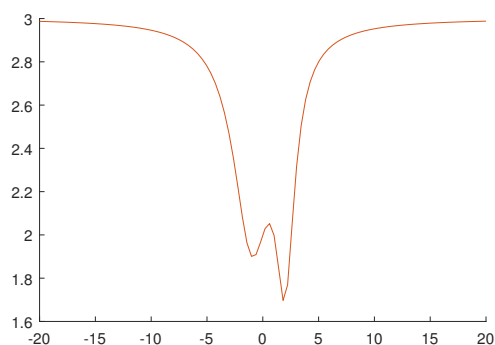
Figura 1: Função objetivo unidimensional para o problema de localização de instalações.
