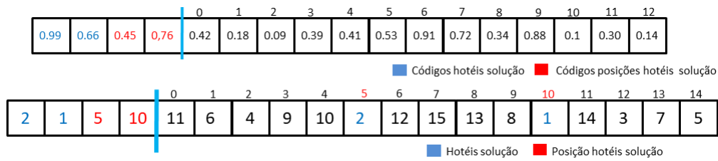
Figura 3: Solução codificada e decodificada com D = 2 .
